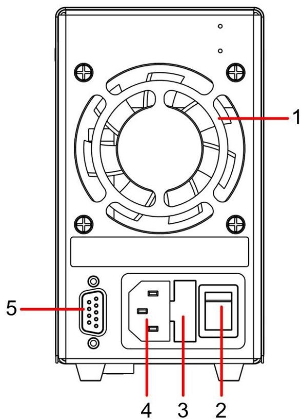
图 2-4 后面板概览（带 RS232 机型）
