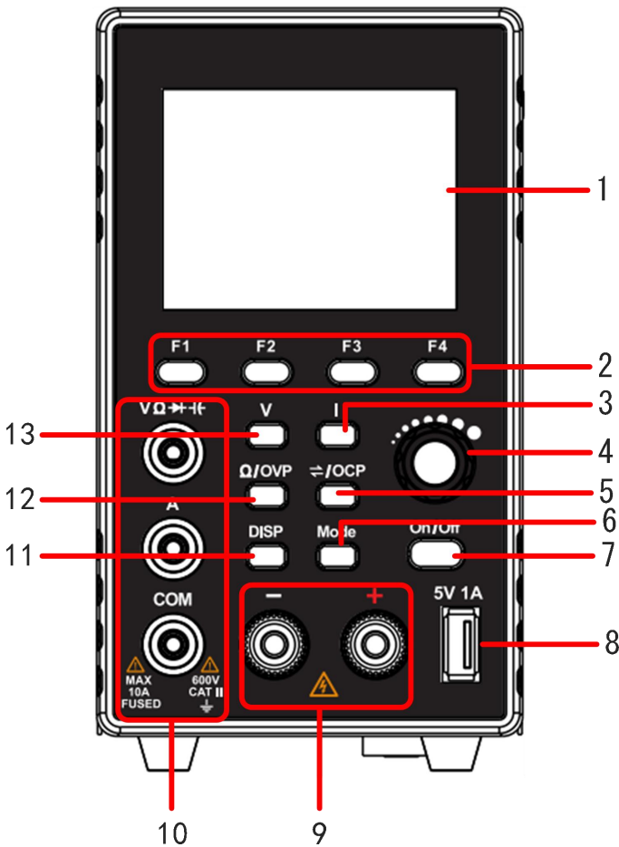
图 2-1 前面板概览
