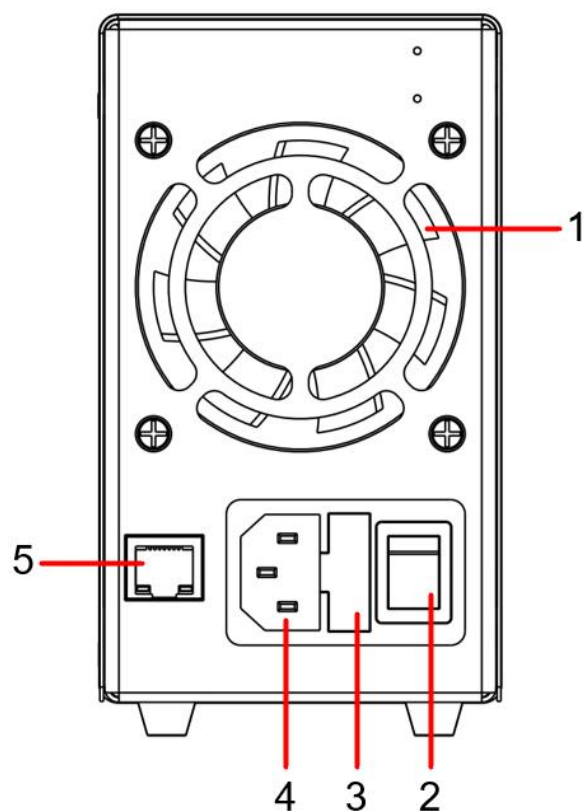
图 2-3 后面板概览（带 LAN 机型）
