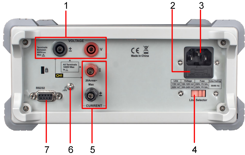
OWH98 单相系列后面板概览
