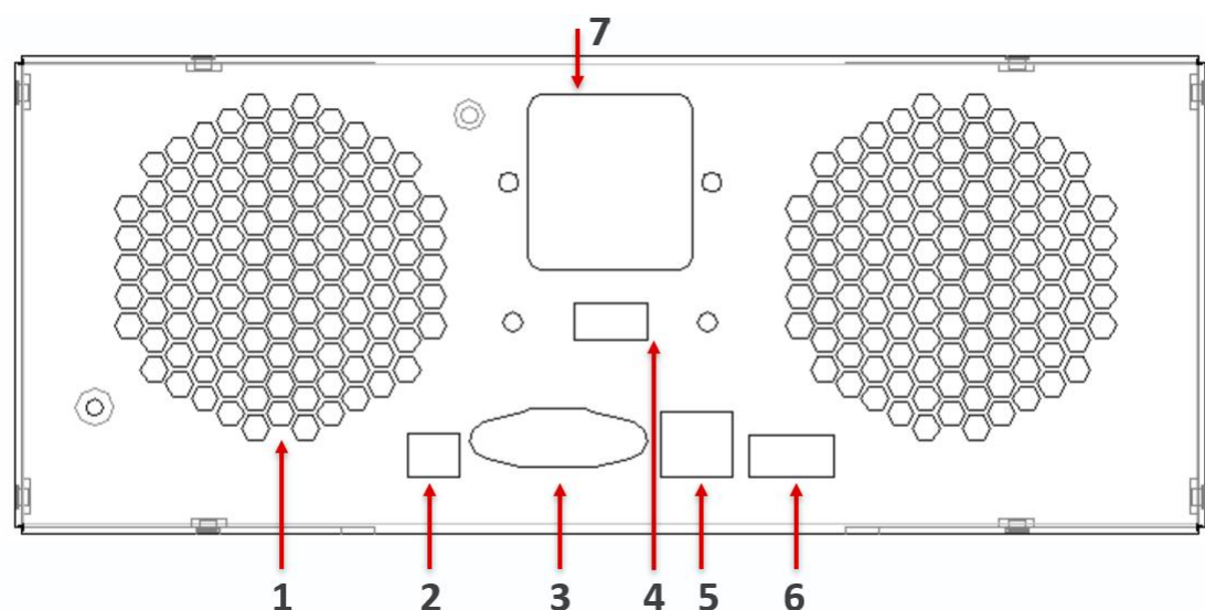
图 3-2 后面板概览
