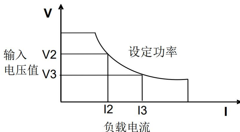
图 4.3.4-1 恒定功率模式 电压电流关系图
