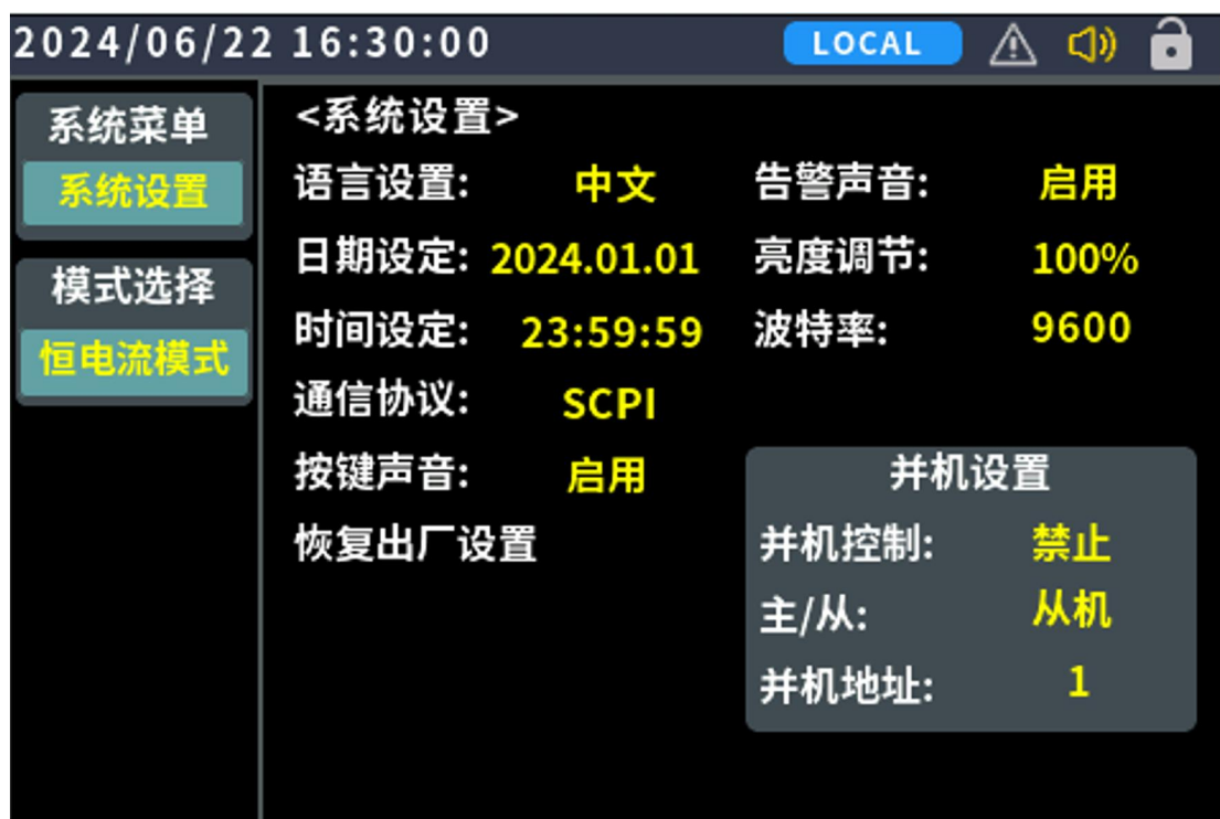
图 4-7-1 系统设置页
