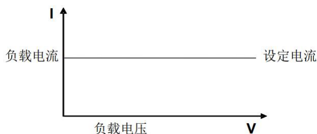
图 4.3.1-1 恒电流模式 电压电流关系图
